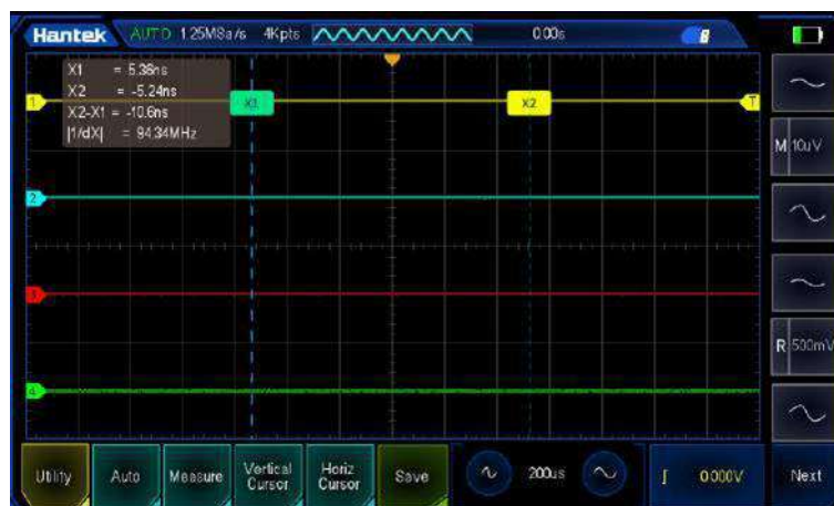
Вертикальные курсоры
