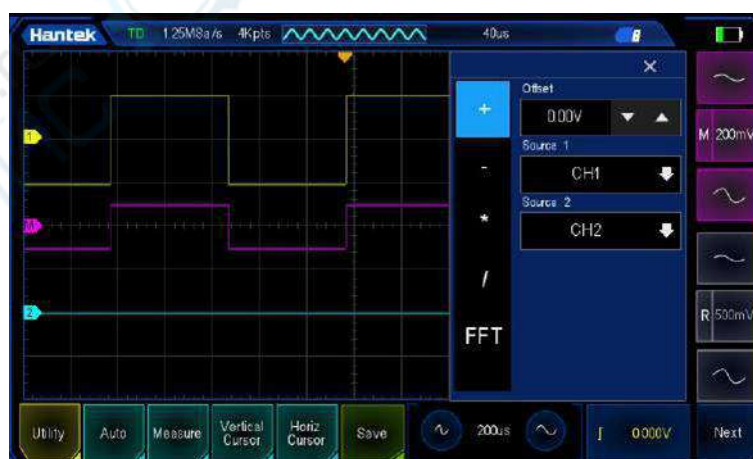
Операция суммирования
