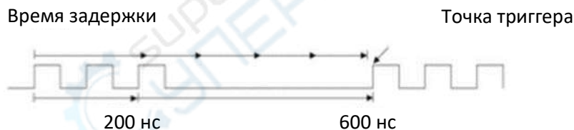
Задержка триггера
